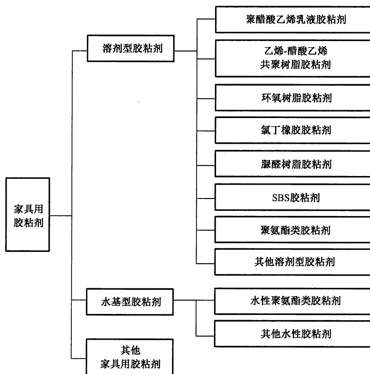
图 9 家具用胶粘剂的分类结构
