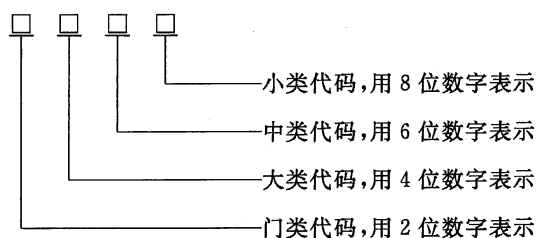
图 1 代码结构图
